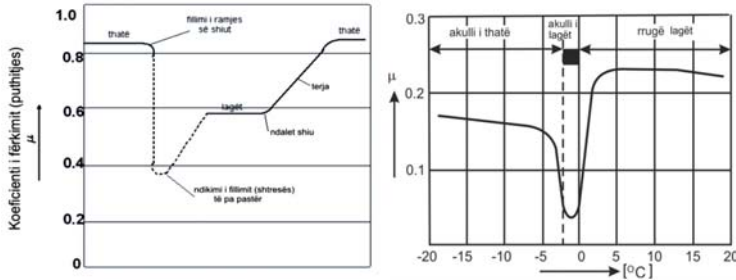
Fig. 7. Koeficienti i ngjitjes në varësi nga gjendja e rrugës dhe temperatura 6
